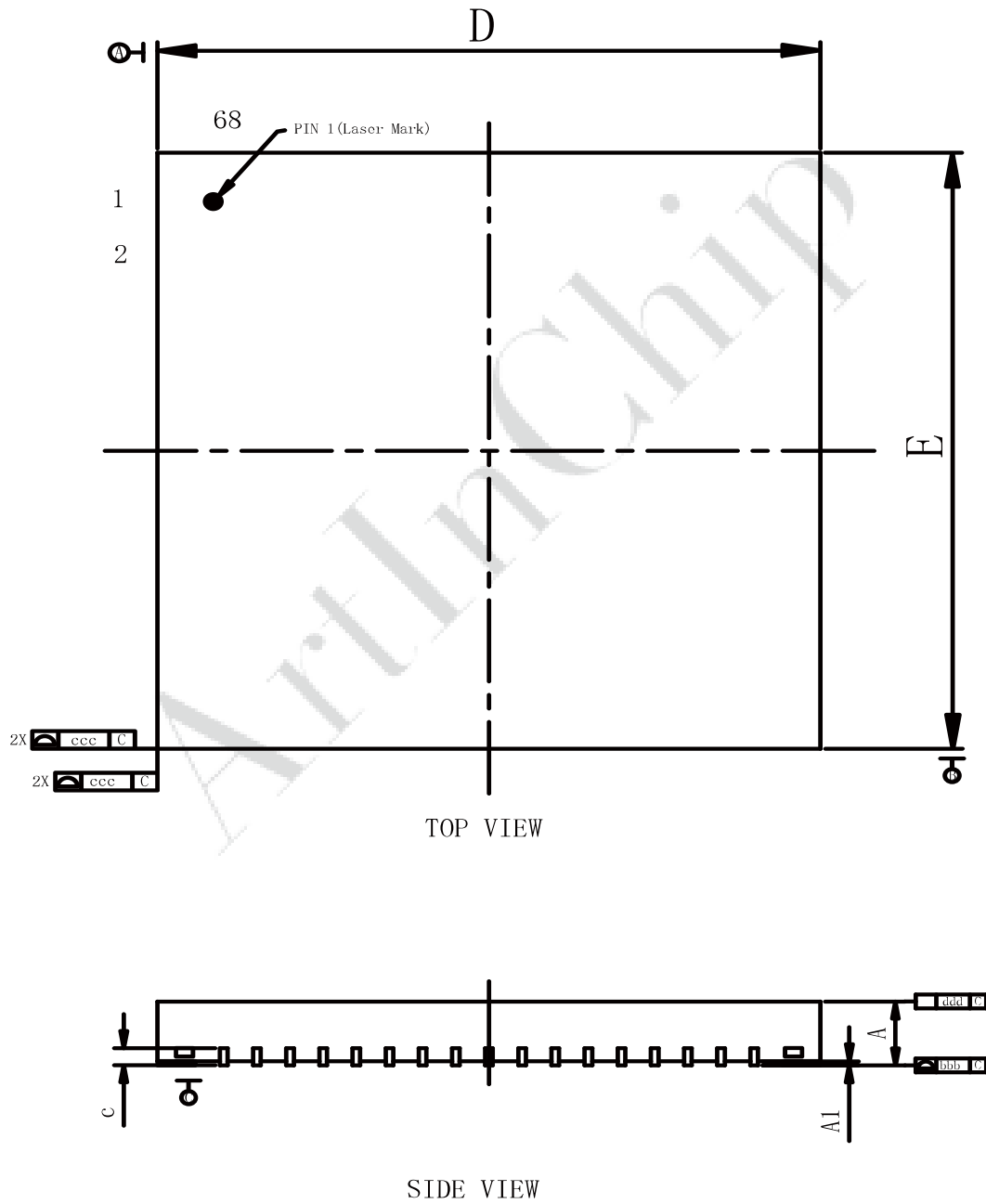
图 5-1 QFN68 封装尺寸图 TOP
